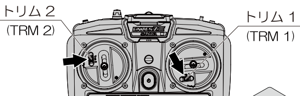
SUB-T設定
