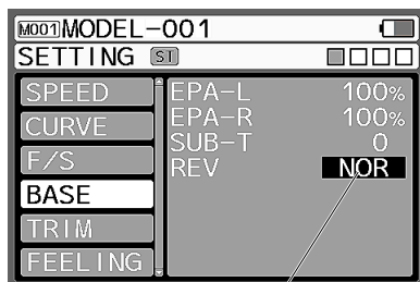
REV設定
